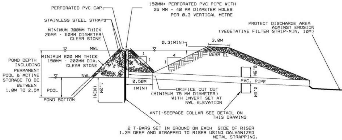
SECTION A-A
